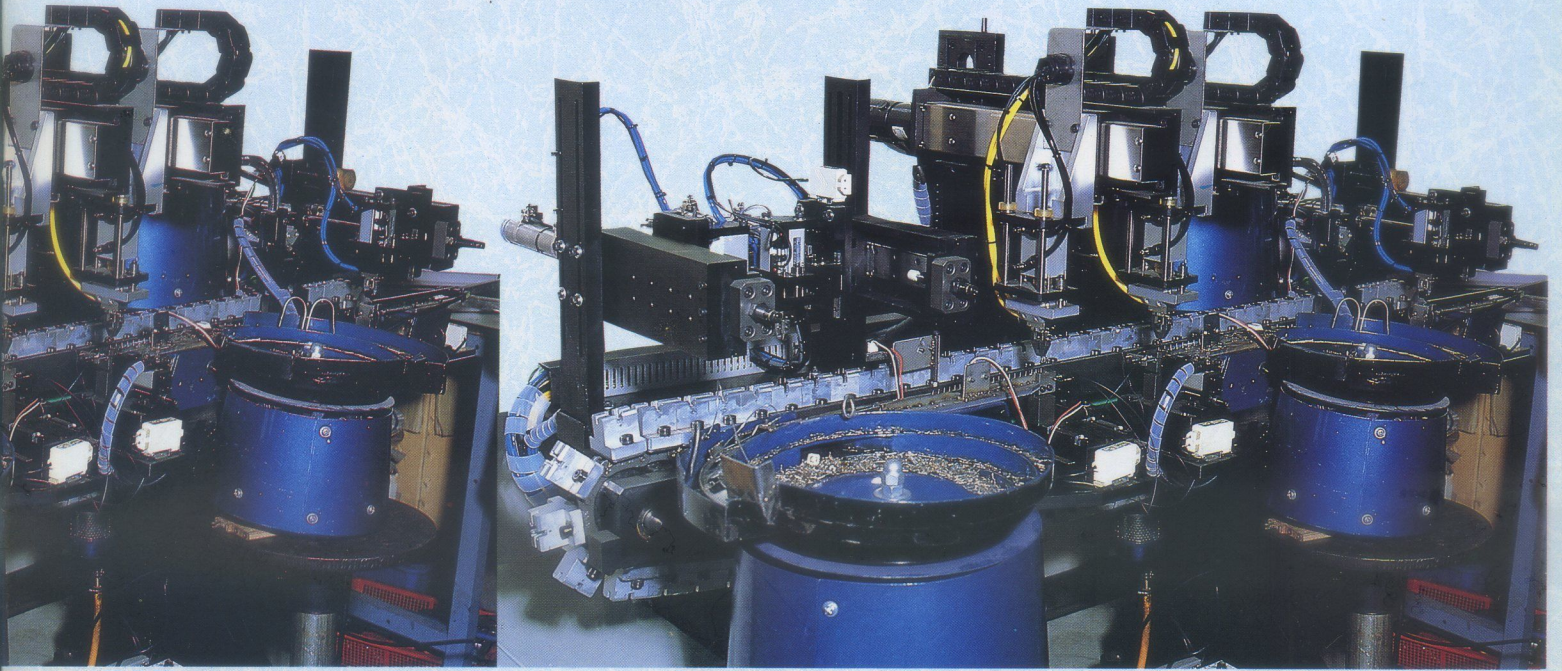
鍵體全自動組裝部份 Fully automatic keyswitch assembly sector
