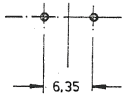
Bohrbild Leiterplatte
